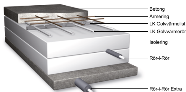
Förläggning av Rör-i-Rör i betongplatta med golvvärme.
