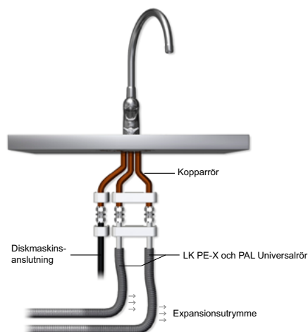
Godtagbar lösning vid installation av köksblandare med anslutningsrör av koppar med LK PE-X och PAL Universälror RiR.
