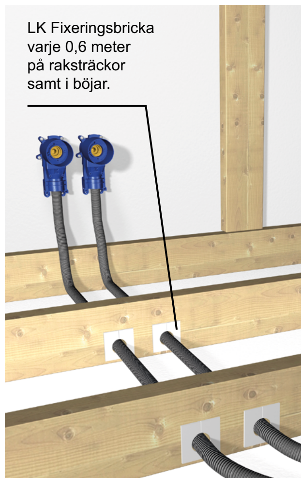
Fixering av Rör-i-Rör i regelkonstruktioner.
